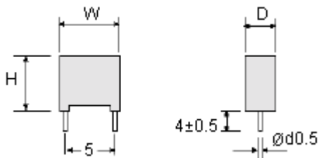
Dimensions : Millimetres
