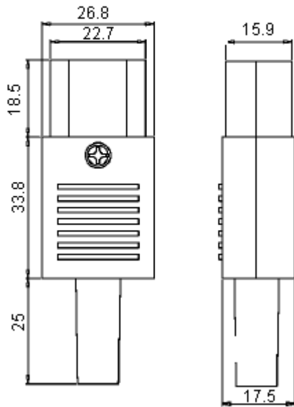
Dimensions : Millimetres
