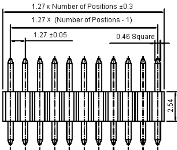
Dimensions : Millimetres
