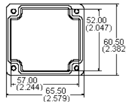
Lid - Inside
