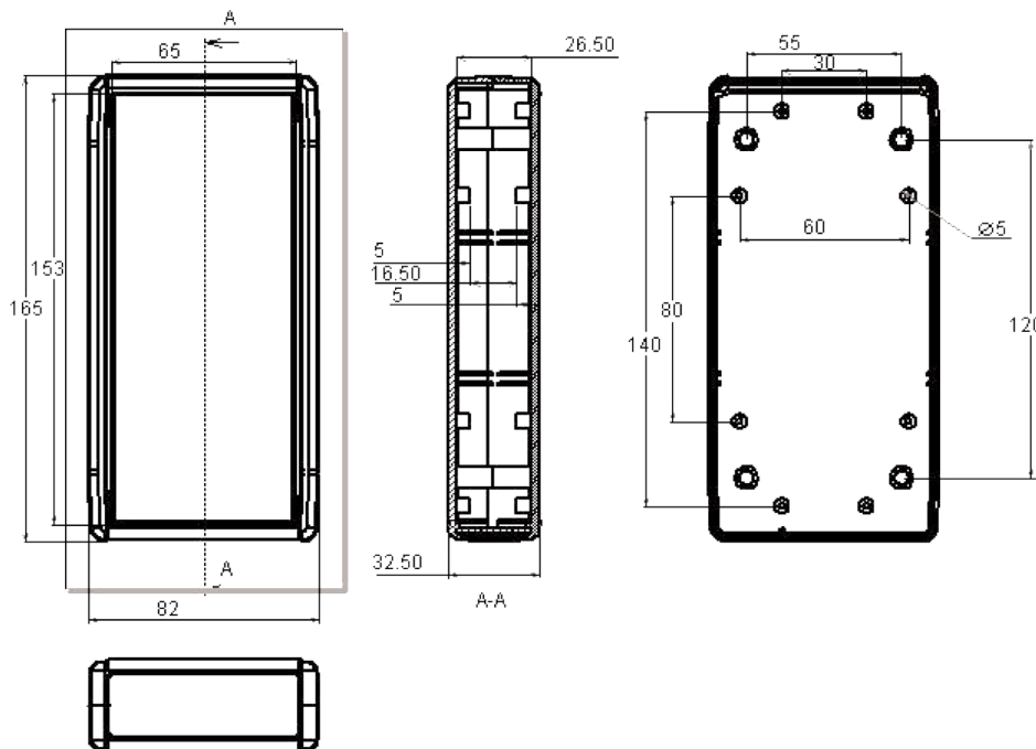
Dimensions : Millimetres
