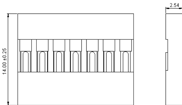
Dimensions : Millimetres
