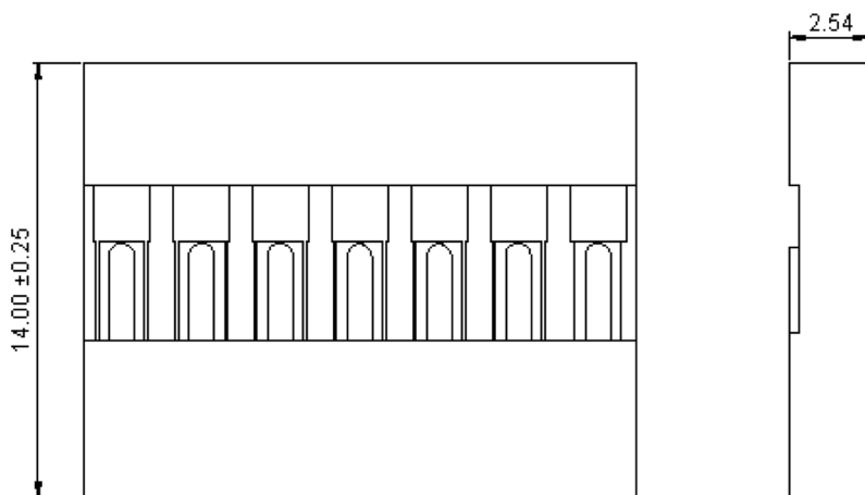
Dimensions : Millimetres
