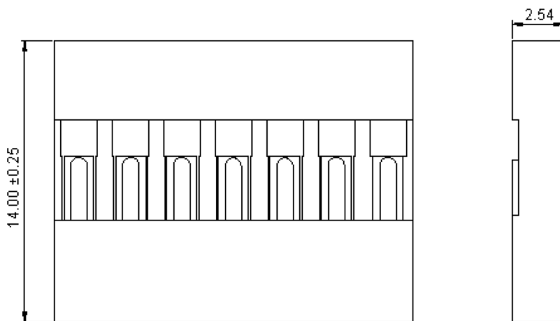
Dimensions : Millimetres
