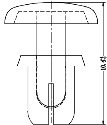
Dimensions : Millimetres
