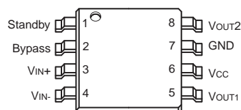
TS4871IQT - DFN8
