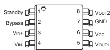
TS4871IST - MiniSO8
