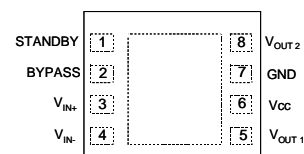
TS4871IQT - DFN8
