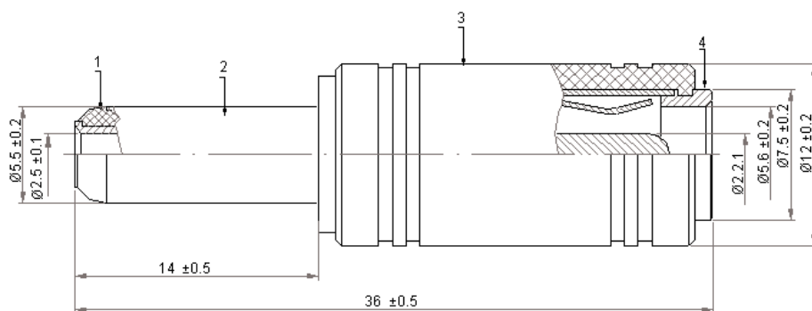
Dimensions : Millimetres
