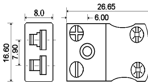
Miniature Socket
