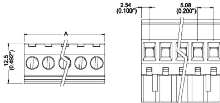
Dimensions : Millimetres (Inches)
