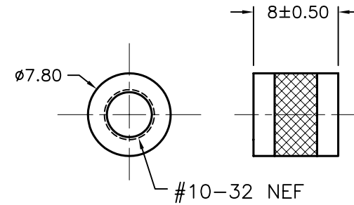
NUT
