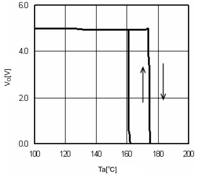
Fig.16 TSD (I o =0mA)
