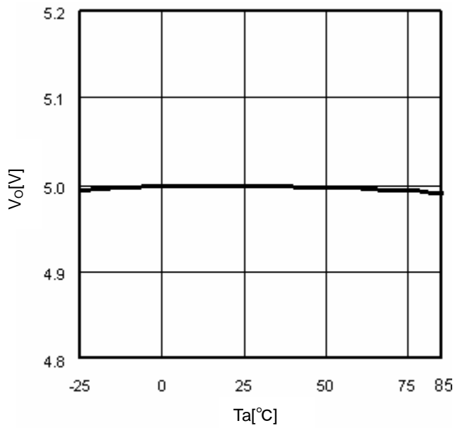
Fig.9 T_a-V_O ( I_o=0mA )
