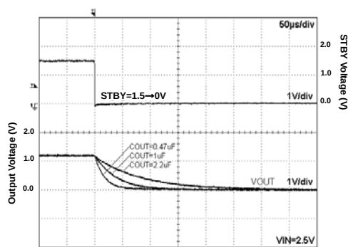
Fig 26. Discharge Time
