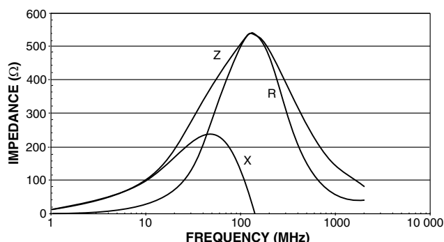
ILHB-0805 600 \Omega
