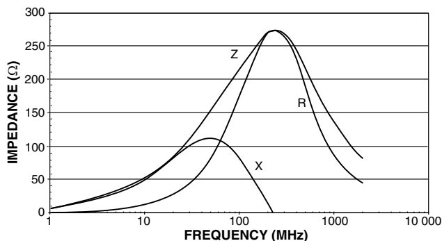
ILHB-0805 250 \Omega
