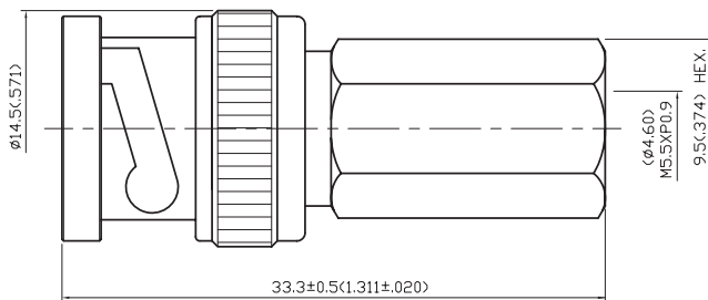
Dimensions : Millimetres (Inches)
