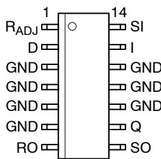
SO-14
