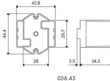
Top 35 mm rail (EN 60715) adaptor for 56.34
