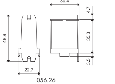
Top 35 mm rail (EN 60715) adaptor for 56.32
