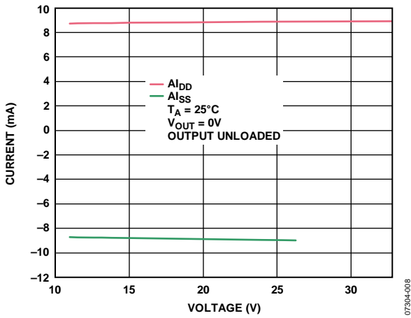
Figure 66. I_{DD}/I_{SS} vs. AV_{DD}/AV_{SS}
