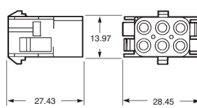
Cap
