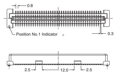
Receptacle
