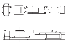
Receptacle Contact
