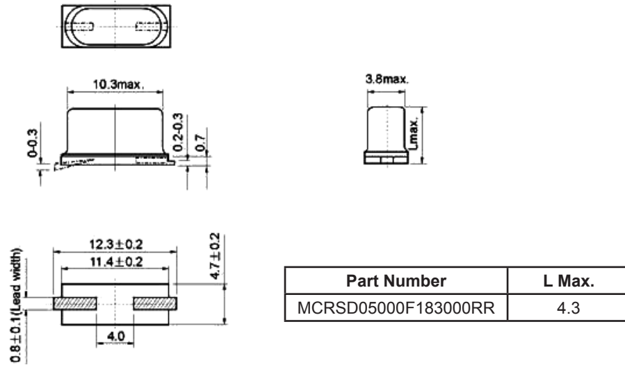
Dimensions : Millimetres
