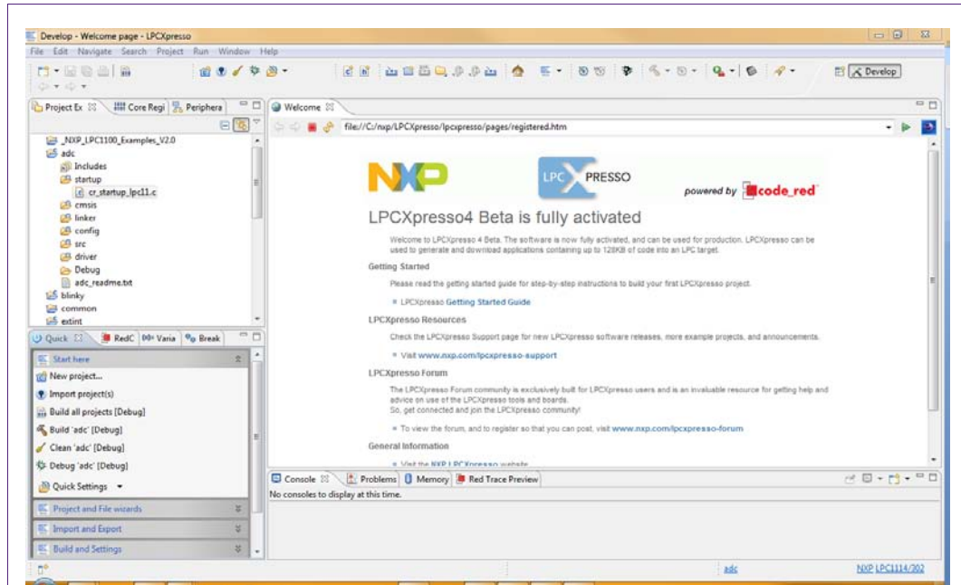
Fig 1. LPCXpresso IDE
