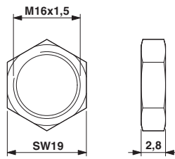
Flat nut M16
