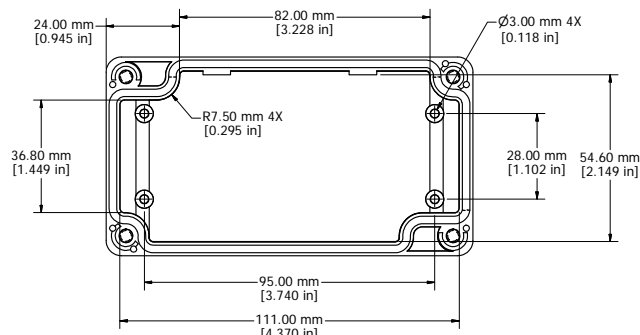
LID - INSIDE
