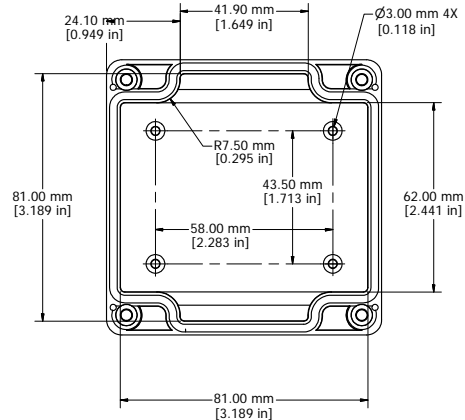
LID - INSIDE
