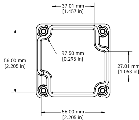
LID - INSIDE
