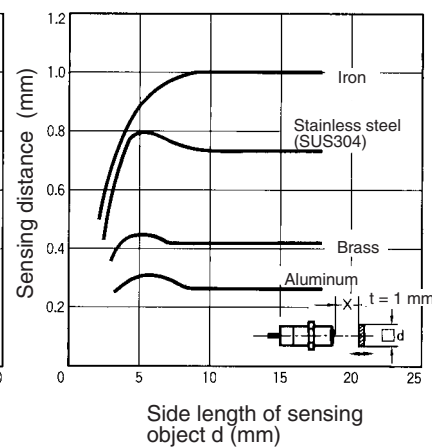
E2E-X1□□ E2E-C1□□
