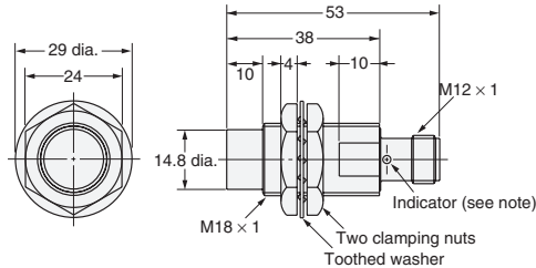
Fig. 24 : E2E-X14MD□-M1(G)/E2E-X10ME□-M1/F□-M1 E2E-X10MY□-M1
