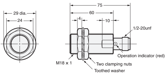
E2E2-X5Y□-M4
