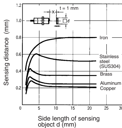
E2E-CR8□□
