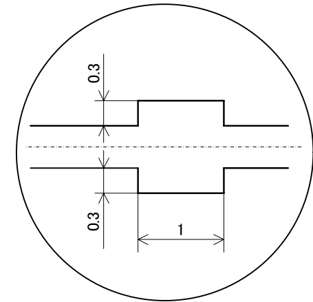
ストッパー部詳細図 Detail of stopper
