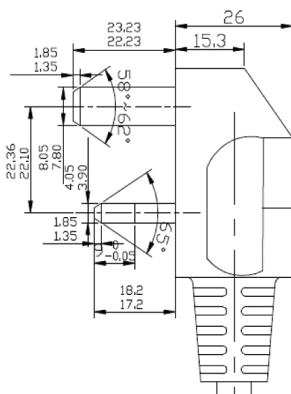
Dimensions : Millimetres
