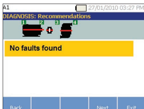
4. Vérification de résultat en utilisant l'outil de test de vibration Fluke.
