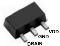
SOT-89 (N8)
