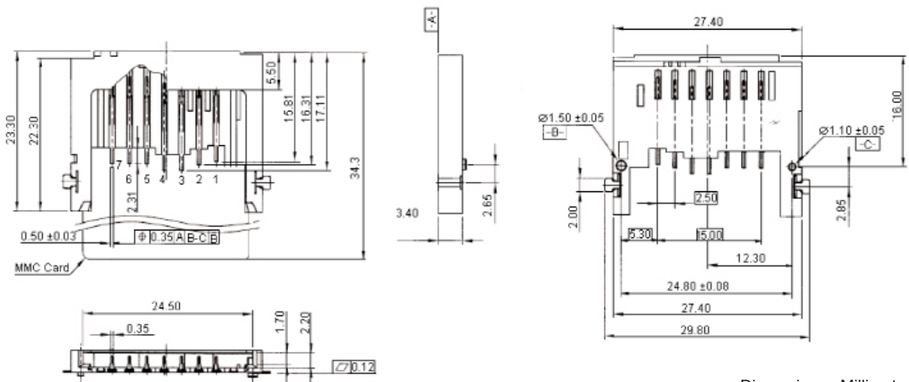
Dimensions : Millimetres
