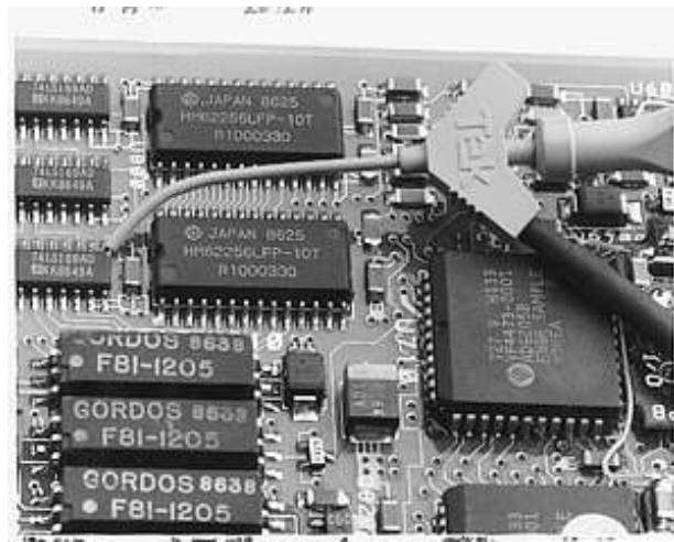
SMT KlipChip Adapter.
