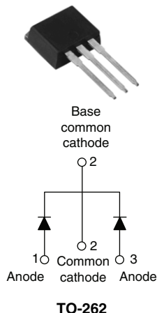
VS-47CTQ020-1PbF
