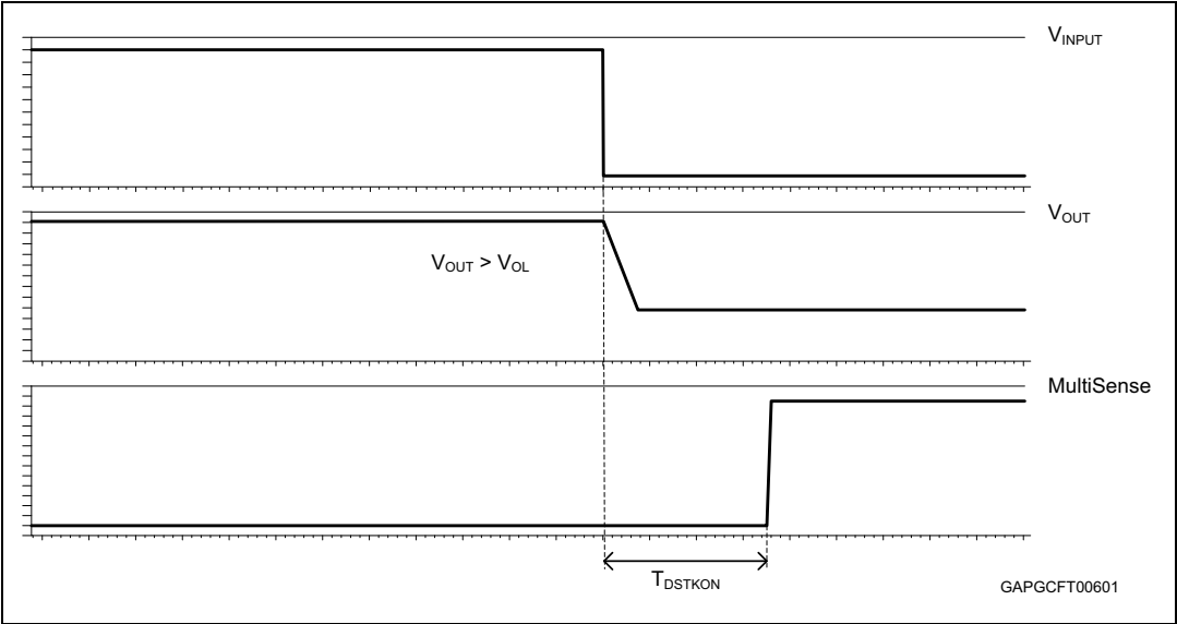
Figure 9. T_{DSTKON}
