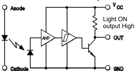
OPB917BZ 10K Pull-Up
