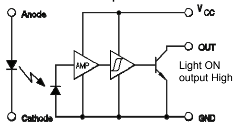
OPB917BOCZ Open-Collector
