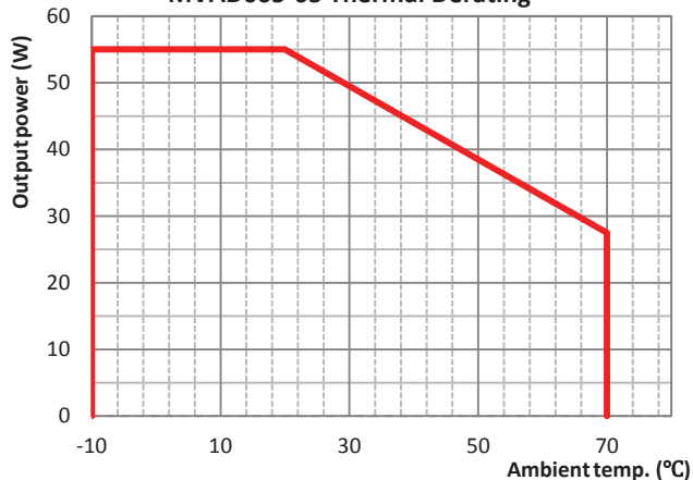
MVAD065-05 Thermal Derating
