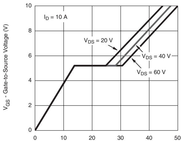
I_D = 10\text{ A} V_{DS} = 20\text{ V} V_{DS} = 40\text{ V} V_{DS} = 60\text{ V} Gate Charge
