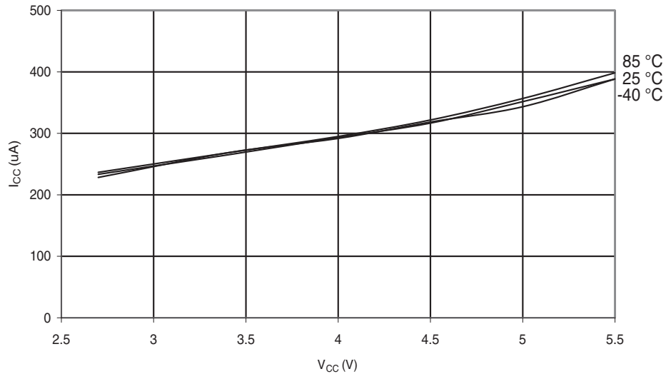
Figure 28-46. ADC Current vs. AV CC (ADC at 50kHz)
