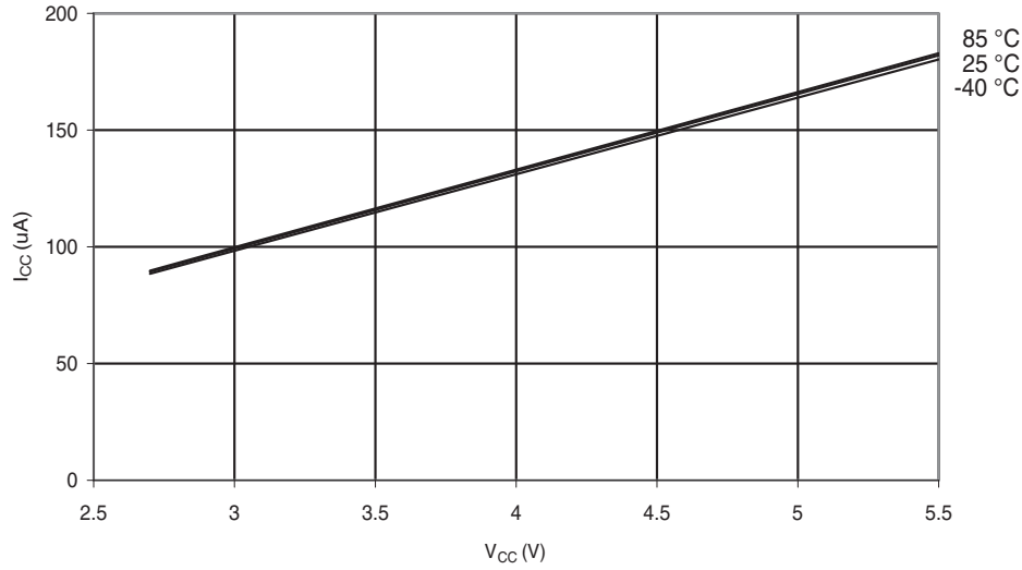
Figure 28-47. ADC Current vs. AV CC (ADC at 1MHz)
