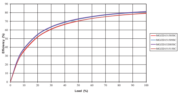
15V INPUT
