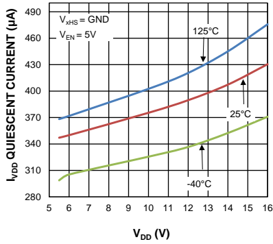
V DD Quiescent Current vs. V DD Voltage
