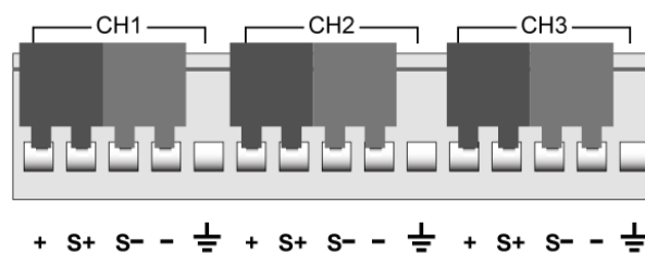
Schéma 18- Jumpers installés pour la régulation locale
