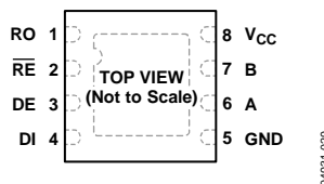
ADM4850/ADM4852/ADM4853
