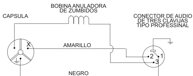
CONEXIONES INTERNAS FIGURA 2
