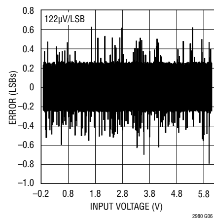
ADC DNL
