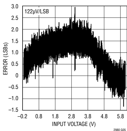
ADC INL
