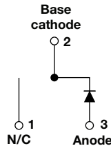
TO-263AB (D²PAK)
