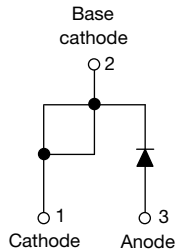
TO-220AC
