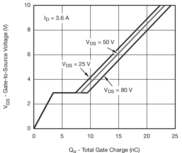
I_D = 3.6 A V_{DS} = 50 V V_{DS} = 25 V V_{DS} = 80 V Gate Charge
